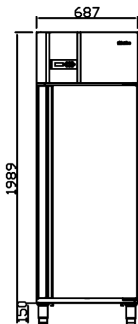
ALZADO
