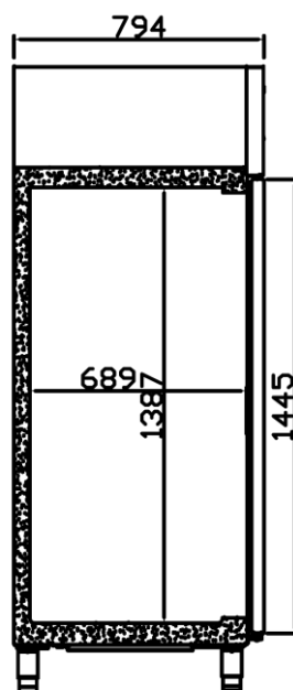
PERFIL
