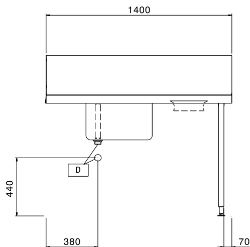
Alzado
