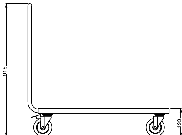
Alzado
