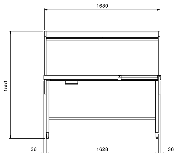
Alzado
