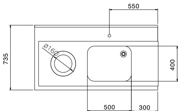
Planta
