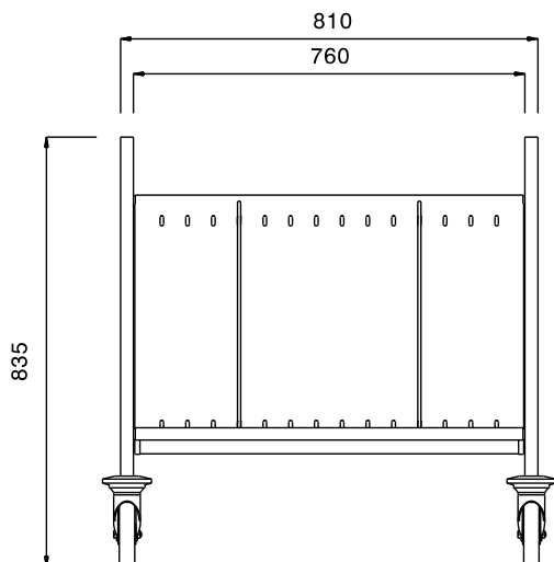
Alzado
