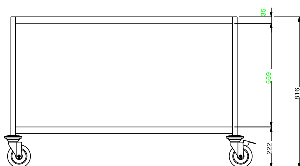
Alzado
