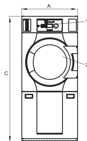
Frontal
