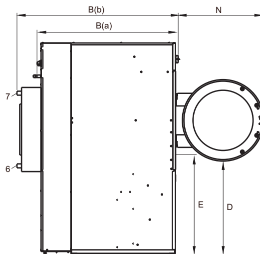
Lateral izquierdo
