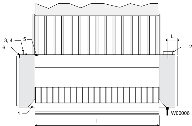
Vista superior
