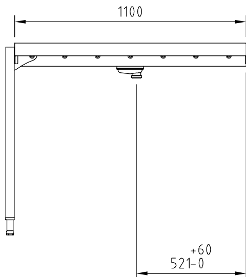
Alzado
